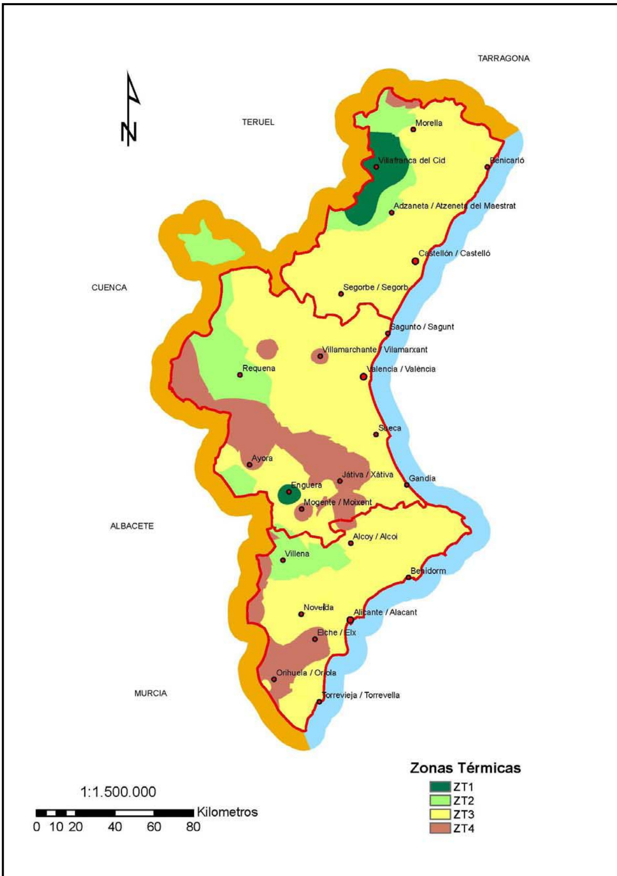
Figura 1 - Zonas térmicas de la Comunitat Valenciana
