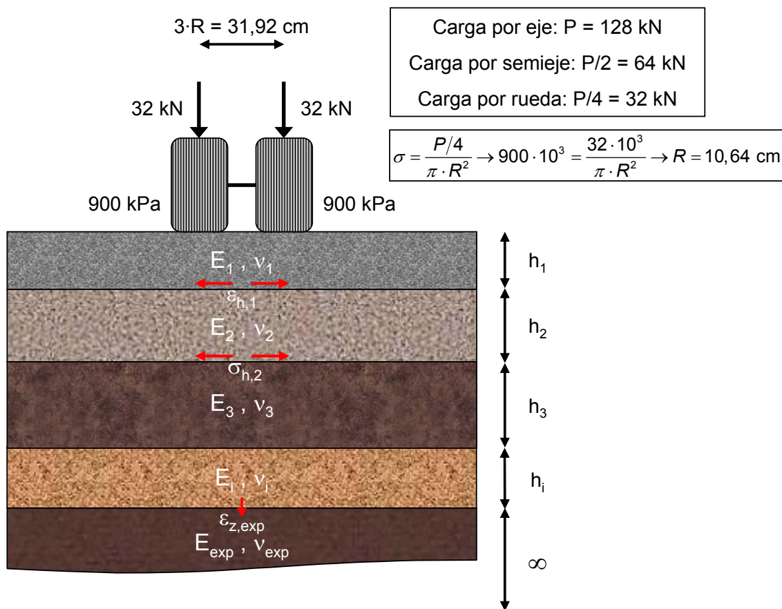
Figura 3 - Esquema de carga y sección tipo
