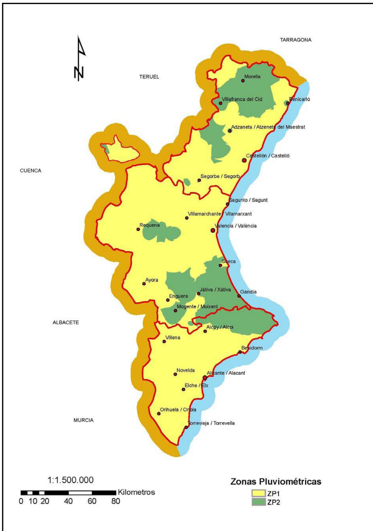
Figura 2 - Zonas pluviométricas de la Comunitat Valenciana
