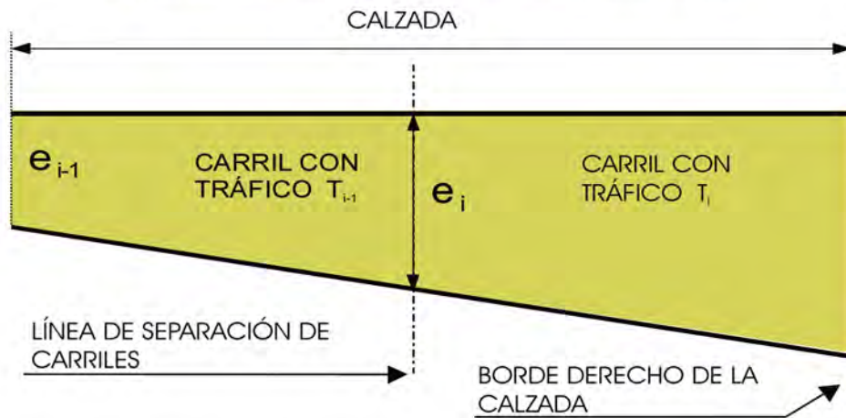
Figura 12. 2 Esquema de variación de espesor entre carriles
